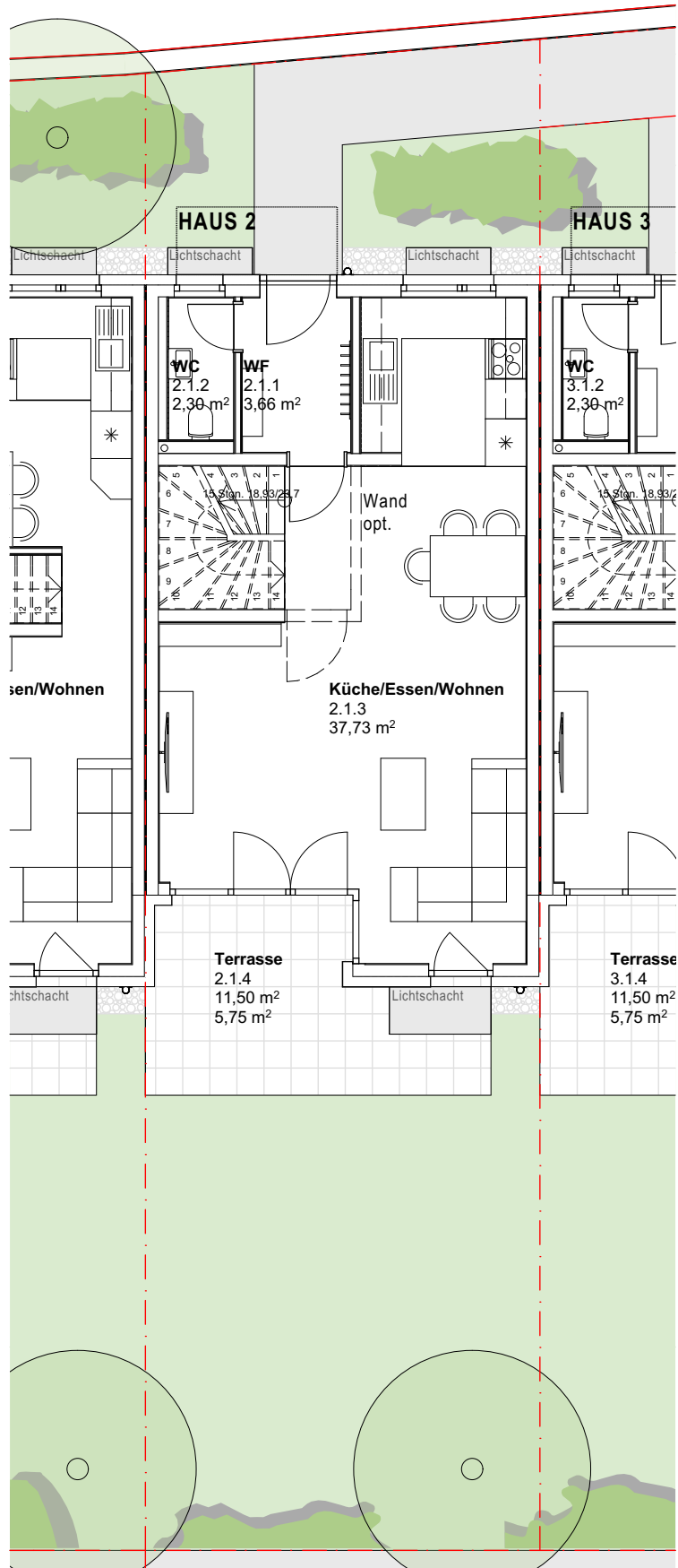
ERDGESCHOSS Haus 2 M 1//100
