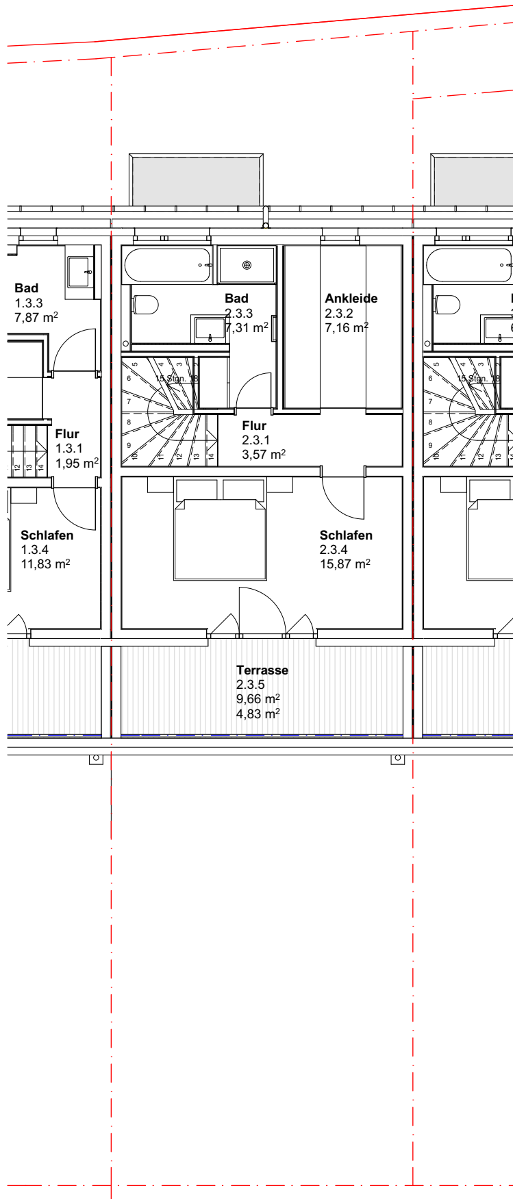
DACHGESCHOSS Haus 2 M 1/100
