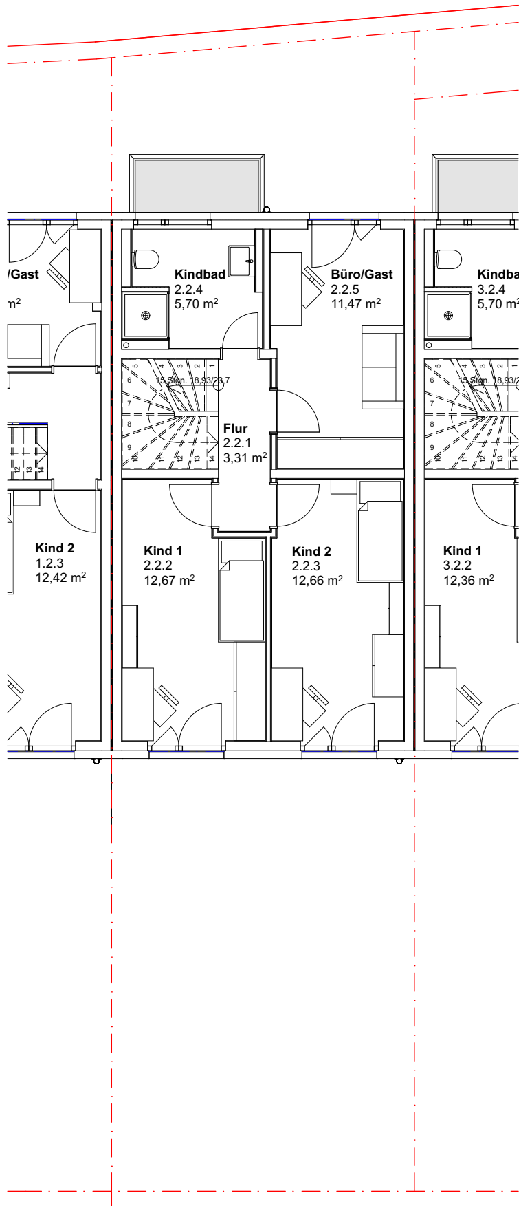
OBERGESCHOSS Haus 2 M 1//100
