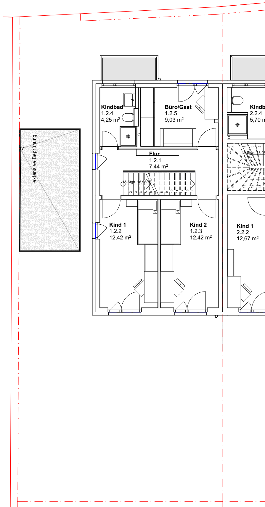
OBERGECHOSS Haus 1 M 1//100
