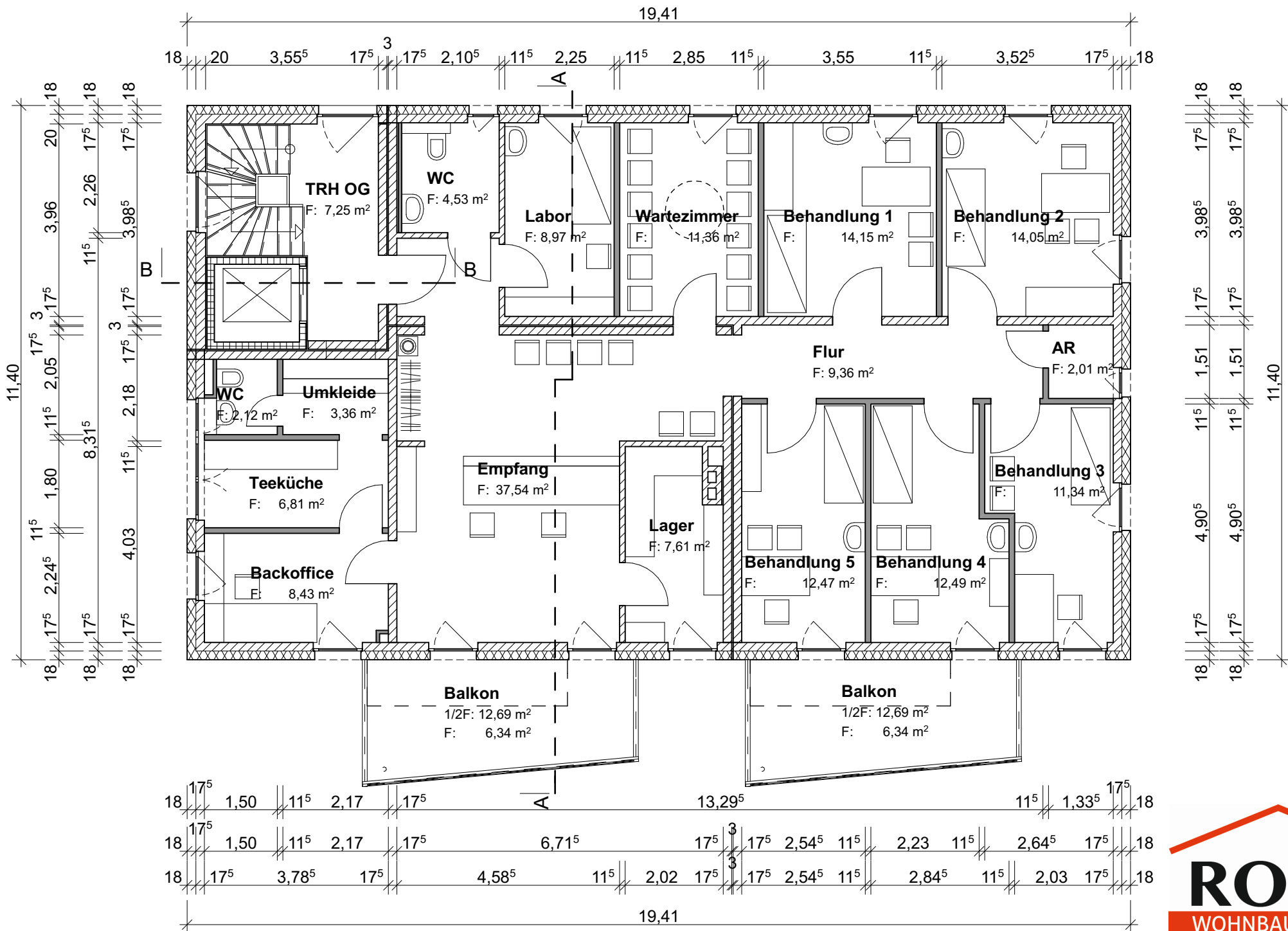
Grundriss Obergeschoss M 1/100
